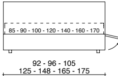
FASCIA APRIBILE DX - SX PER INSERIMENTO 2° LETTO ESTRAIBILE O CASSETTONI L-R OPENABLE BED SURROUND FOR FITTING A 2ND PULL-OUT BED OR STORAGE DRAWERS
